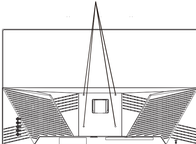
壁掛け金具取り付け用ネジ穴
